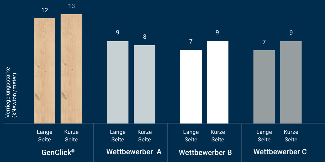
GRAFIK 1: VERRIEGELUNGSSYSTEM (ISO 10582) HÖHERER WERT FÜR DIE VERRIEGELUNGSSTÄRKE = STÄRKERE VERBINDUNG
